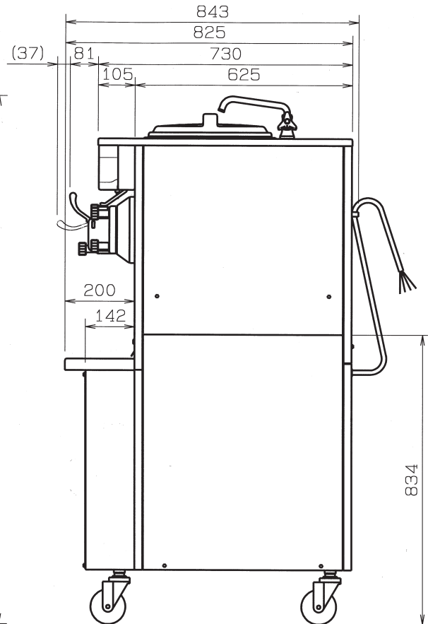
●側面図
