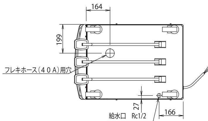
●底面図
